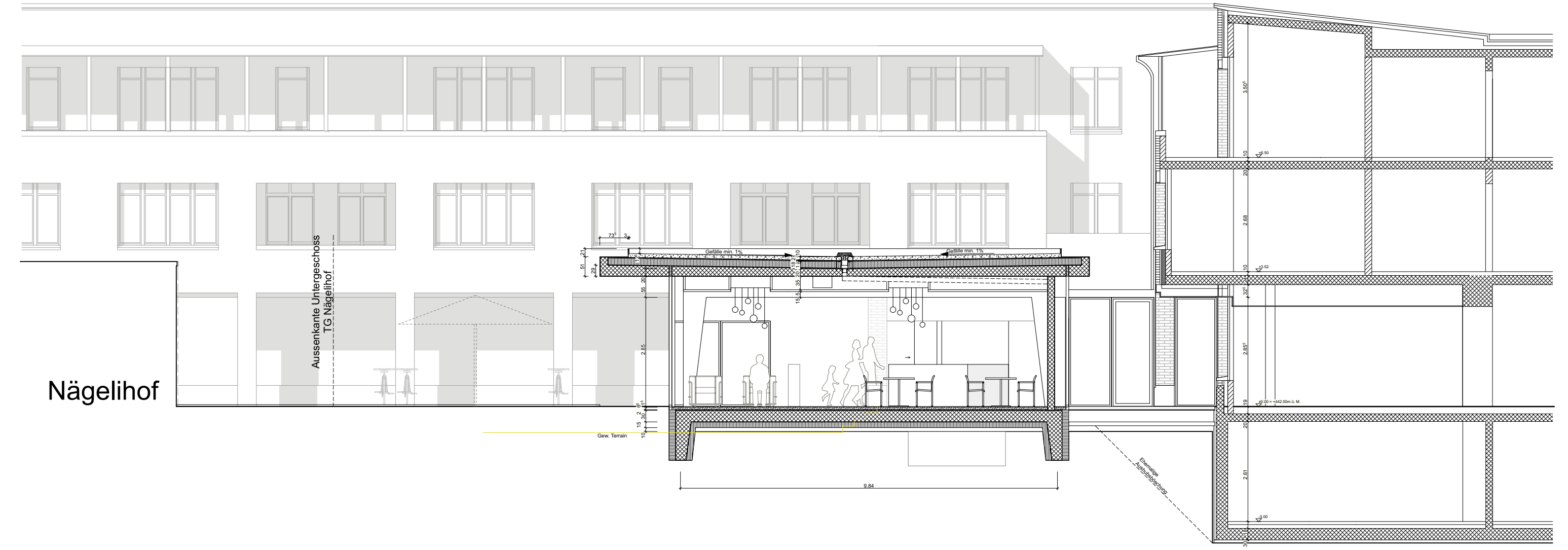
Schnitt 2
