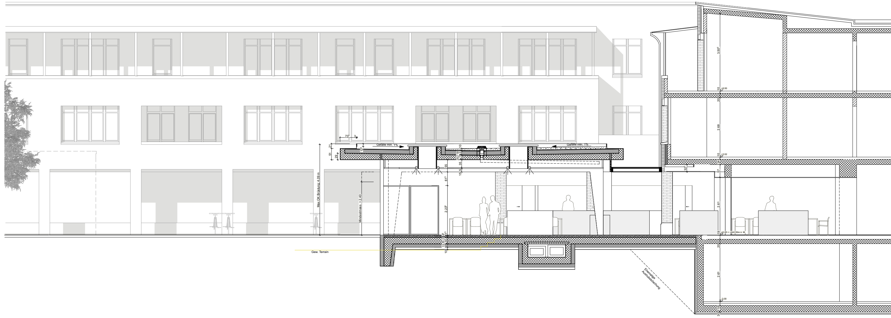
Schnitt 1
